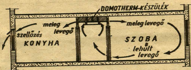
A Domotherm-fűtés működésének vázlata
